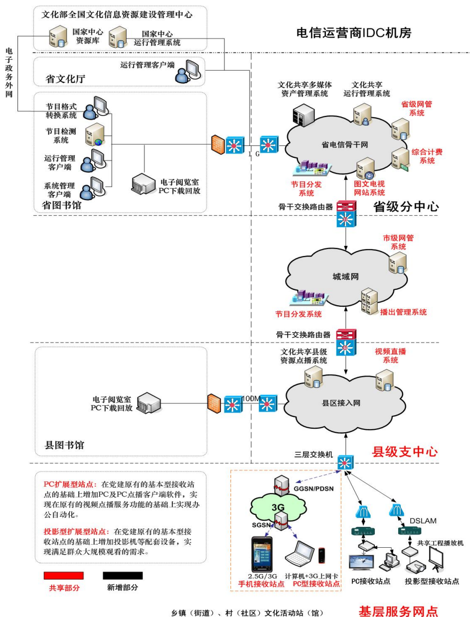
圖 1. 河南省文化信息資源共享工程網絡結構圖 Figure 1. Henan cultural information resources sharing project network structure
